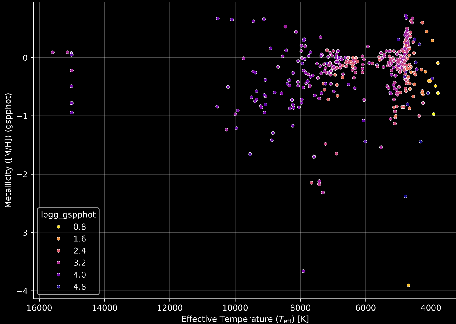
APOGEE DR17 Field: [281+00] Stellar Population Parameters (n= 410)
