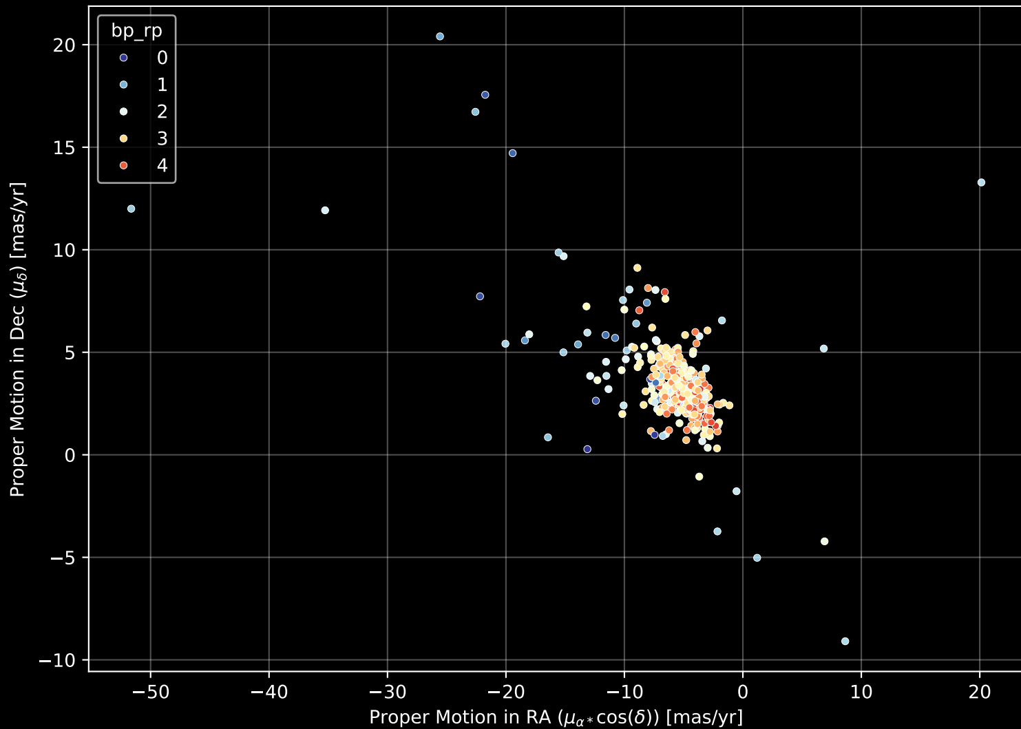
APOGEE DR17 Field: [281+00] Proper Motion Diagram (n= 410)
