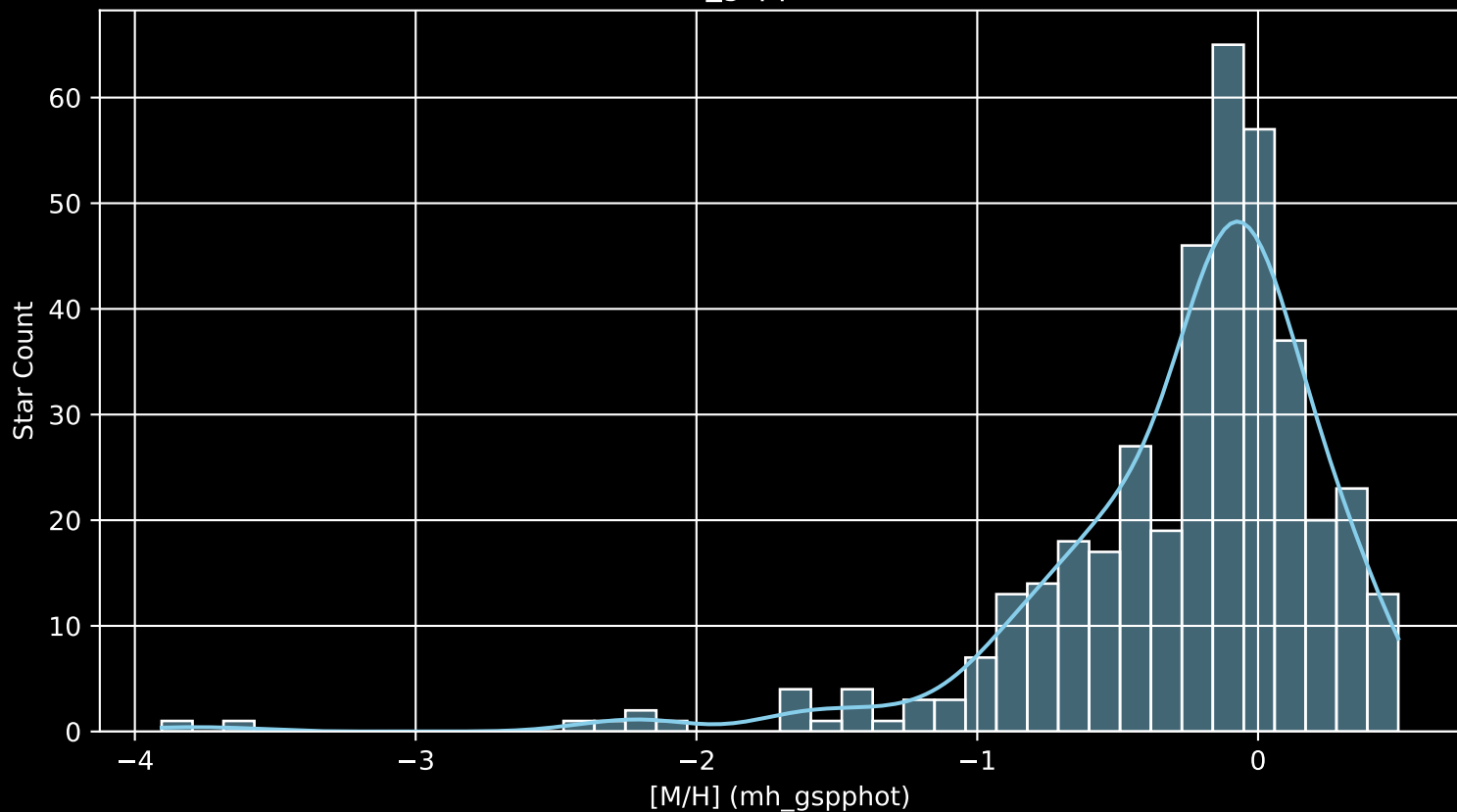
APOGEE DR17 Field: [281+00 [M/H] (mh_gspphot) (n= 399)
